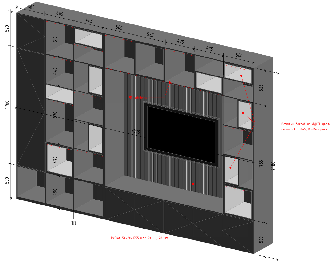
Эскиз настенного стеллажа
