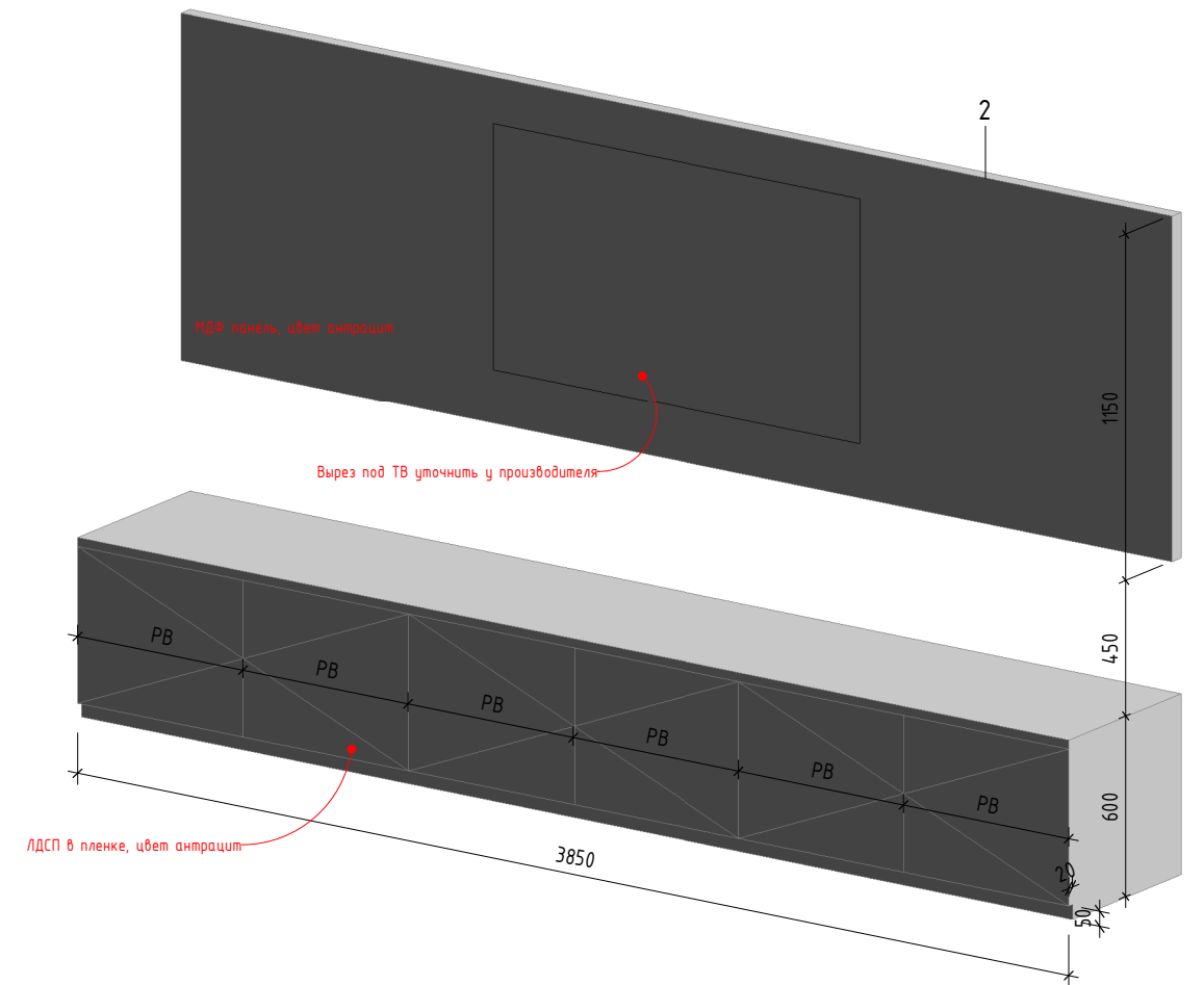
Эскиз тумбы и настенной панели
